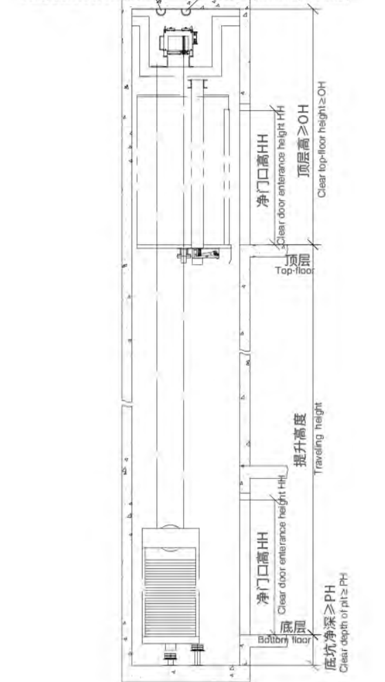
井道立面图 Shaft elevation
