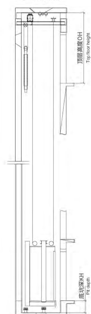
井道立面图 Shaft elevation
