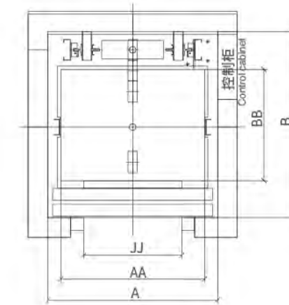
井道平面图 Shaft layout
